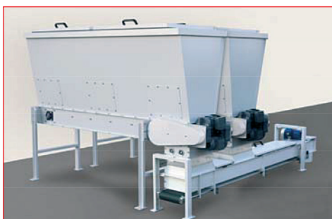
Faserdosiermaschine FS 1000/400
